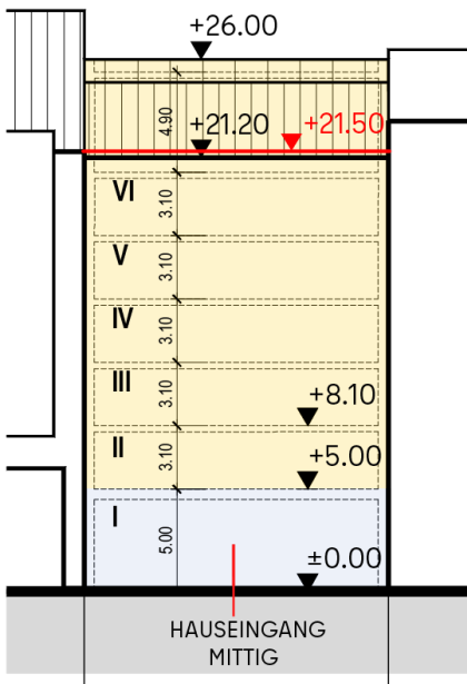
Abb. 7 Schematische Ansicht Haus B 1.3
