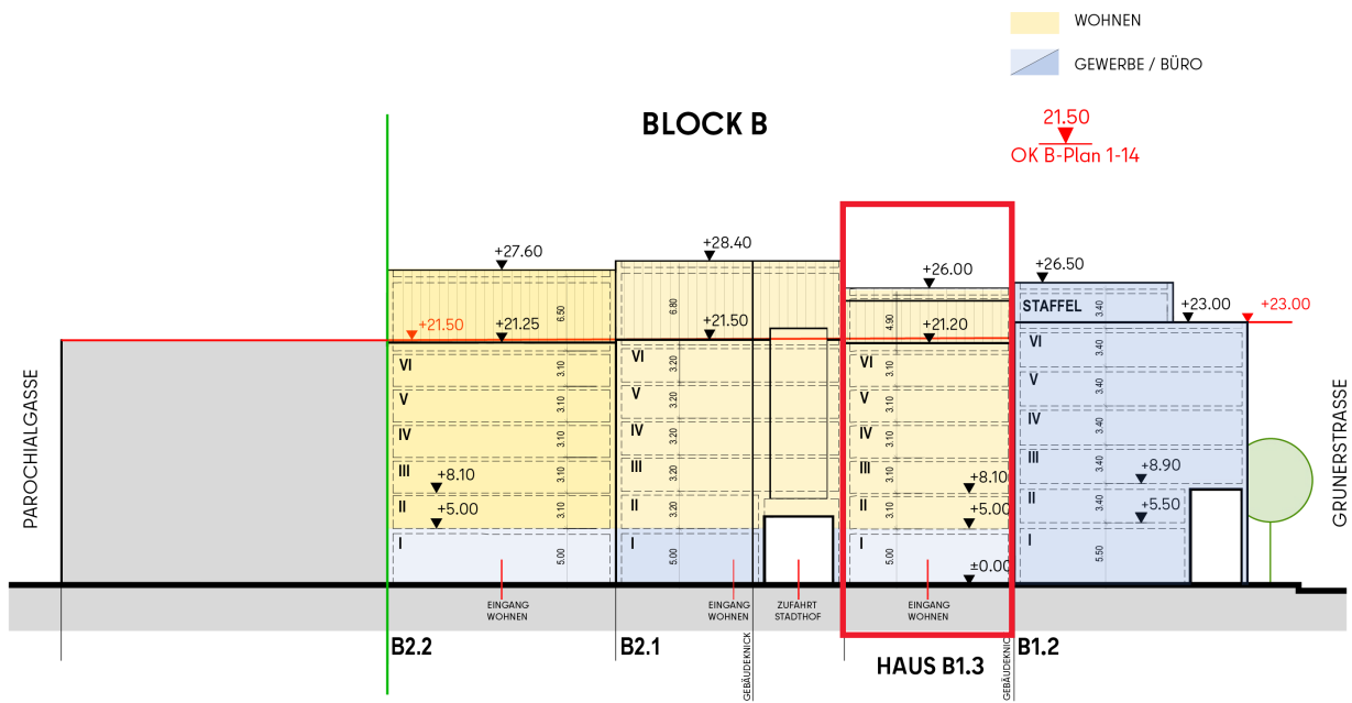
Abb. 6 Schematische Ansicht Judenstraße
