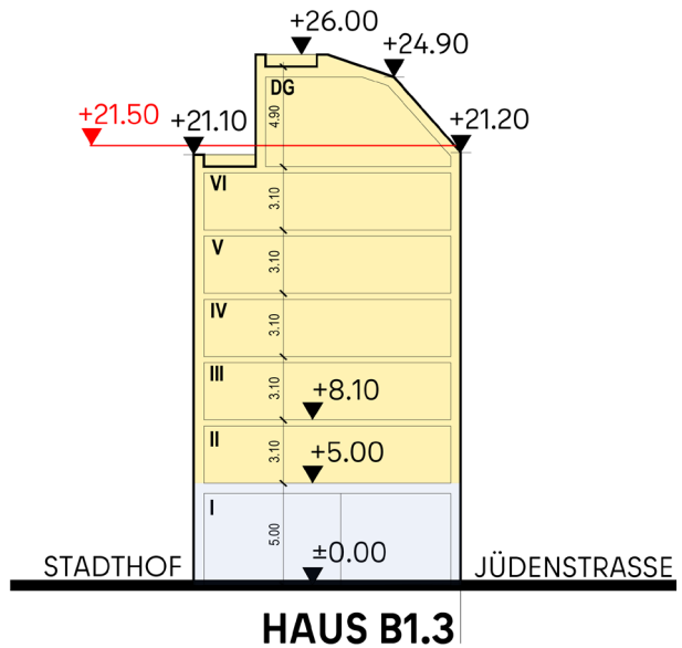
Abb. 8 Schematischer Querschnitt Haus B 1.3
