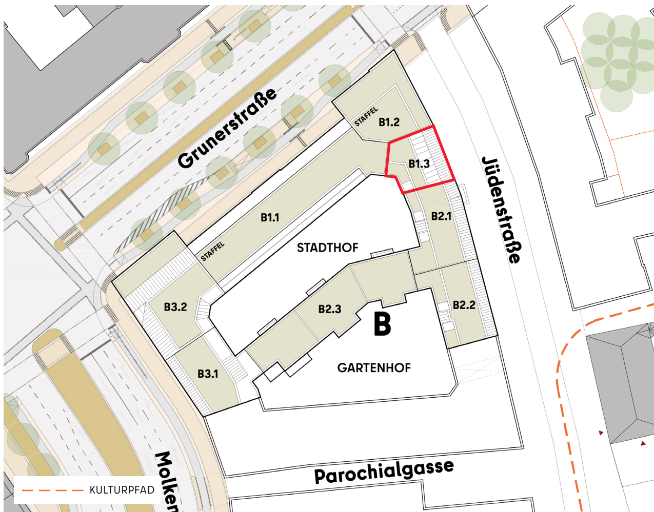
Abb. 1 Dachaufsicht Block B mit Lage Haus B 1.3
