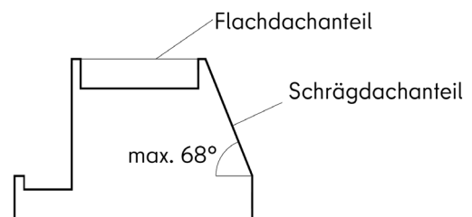
Abb. 5 Schematische Darstellung „Berliner Dach“
