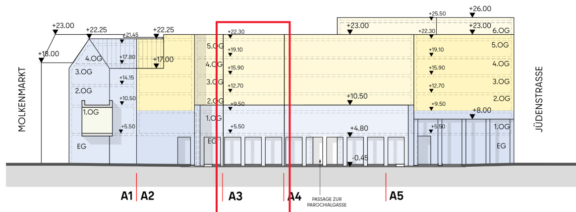
Abb. 9 Schematische Ansicht Stadtplatz-Nord
