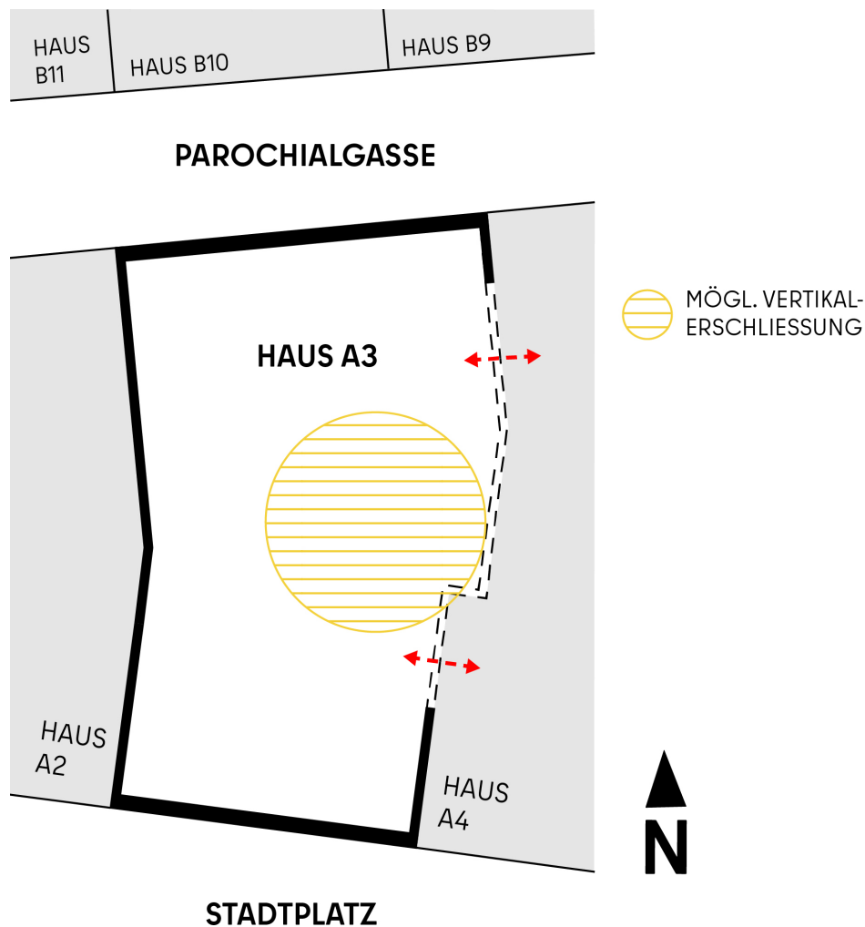
Abb. 4 Schematischer Grundriss Untergeschoss
