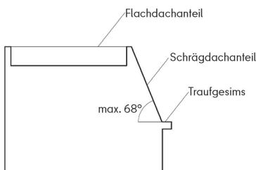
Abb. 11 Schematische Darstellung „Berliner Dach“
