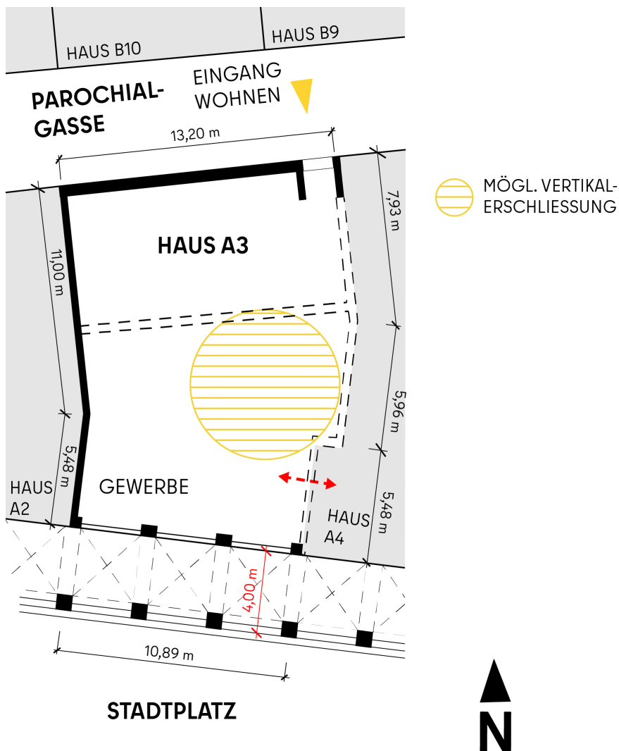
Abb. 2 Schematischer Grundriss Erdgeschoss
