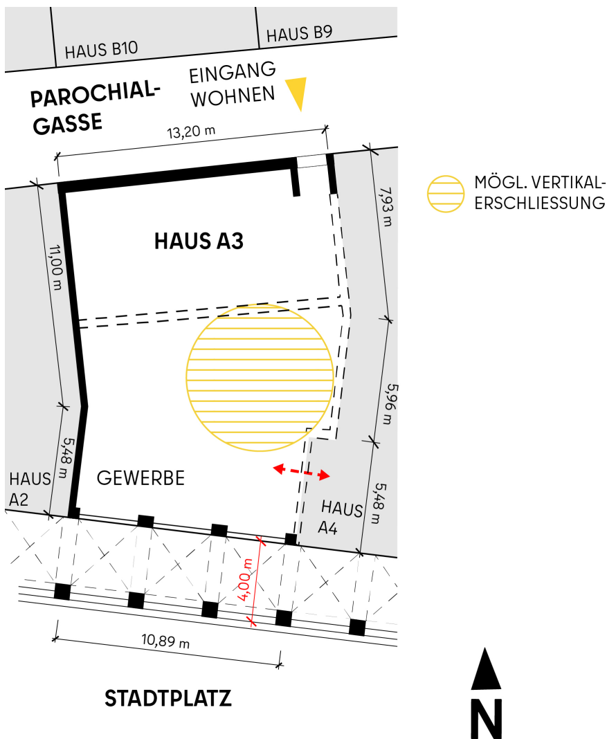
Abb. 5 Schematischer Grundriss Erdgeschoss
